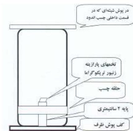
شکل ۱- تصویر شماتیک سیلندرهای آزمایشی مورد استفاده در آزمون پرواز زنبورهای تریکوگراما
